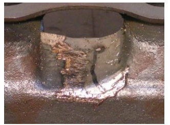
Risse lasergeschweißt
