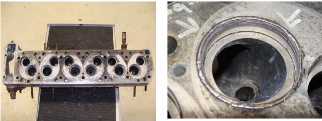
Formel 2, 4 Zylinder, lasergeschweißt
