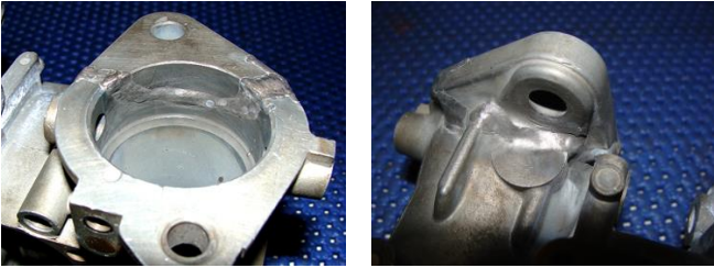
Mercedes 190 SL Vergaser lasergeschweißt
