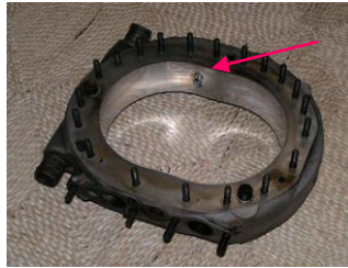
direkt an Chromschicht lasergeschweißt
