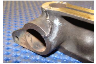
Maybach Kipphebelbrücke lasergeschweißt
